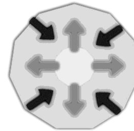
איור 7. שיווי משקל בין כוחות הכבידה פנימה ולחץ מהאנרגיה הגרעינית כלפי חוץ מייצבים את הכוכב
