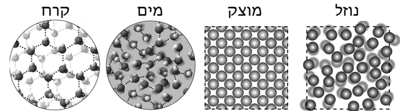
בד"כ חומר במצב מוצק צפוף יותר מאשר כשהוא במצב נוזלי המבנה הגבישי של הקרח גורם למרווחים יותר גדולים בין המולקולות בהשוואה למים
