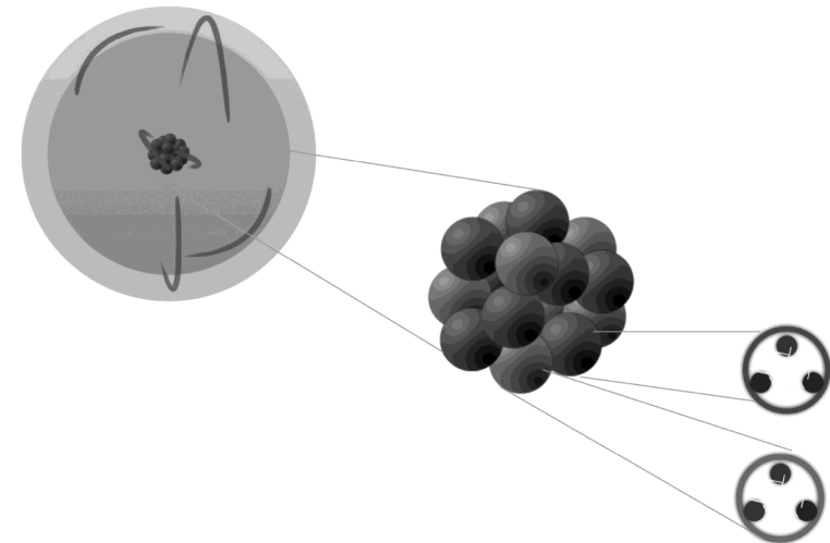
איור 2. לאטום גרעין חיובי ואלקטרונים שליליים. גרעין האטום מורכב מפרוטונים וניטרונים. הפרוטונים והניטרונים מורכבים משלושה קוורקים כל אחד.
